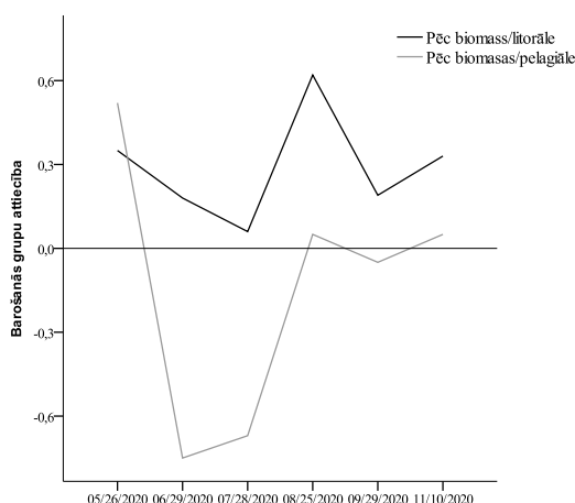
1. attēls. Rotifera barošanās grupu attiecība Saukas ezerā 2020. gada sezonā
